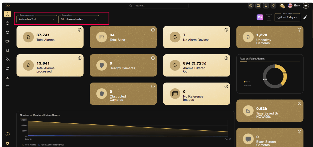
Afbeelding 2: Aangepaste widgetindeling.
